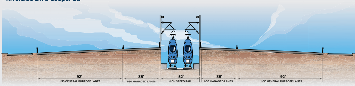
Sección Típica En Trinchera para el Tren de Alta Velocidad en la I-30 Riverside Dr. a Cooper St.
