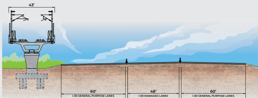
Sección Típica Elevada para el Tren de Alta Velocidad en la I-30 MacArthur Blvd. a Cockrell Hill Rd.
