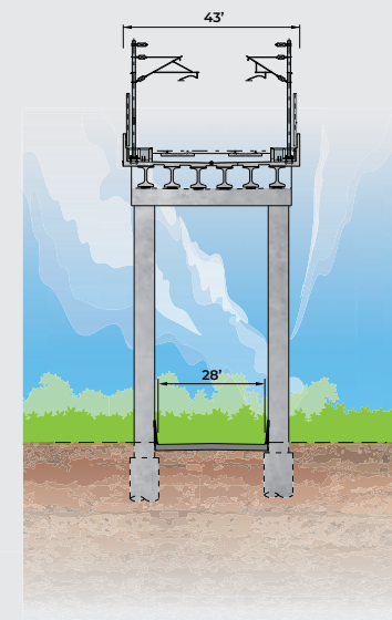
Sección Típica de la Alternativa de Dos Columnas para el Tren de Alta Velocidad en el Centro de Dallas Sobre Hyatt Regency Hotel Dr. y Hotel St.
